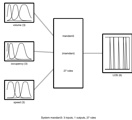
Fig. 6. Mamdani FIS
