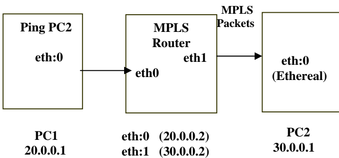
Fig. 6 Test setup
