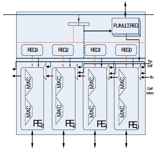
Fig. 4 PU architecture
