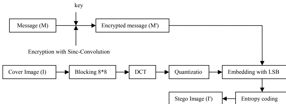
Fig. 1 Encoder
