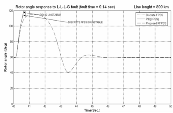
Fig. 10 (d) Fault duration = 0.14 sec.
