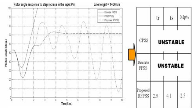
Fig. 8-d L=1400 km
