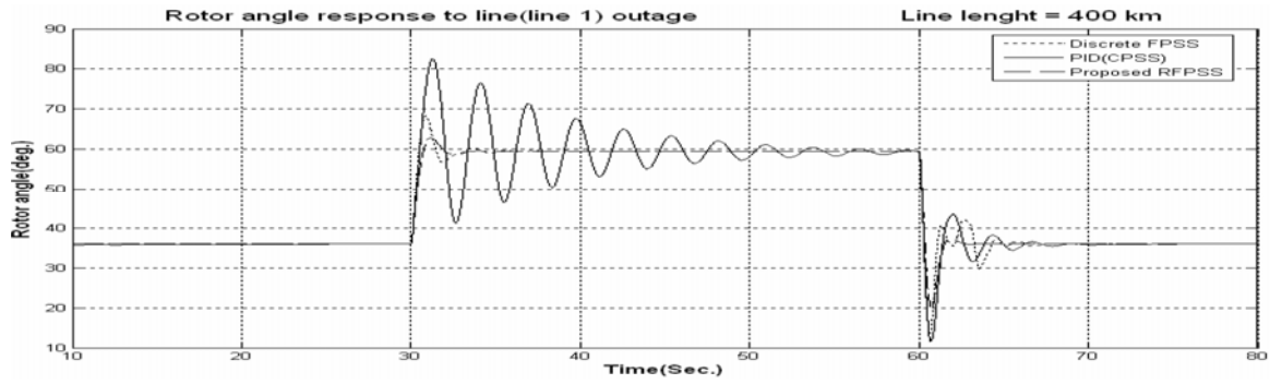
Fig. 9-a L=400 Km
