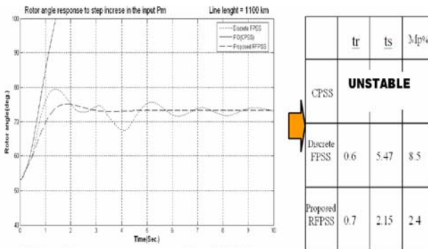
Fig. 8-c L=1100 km
