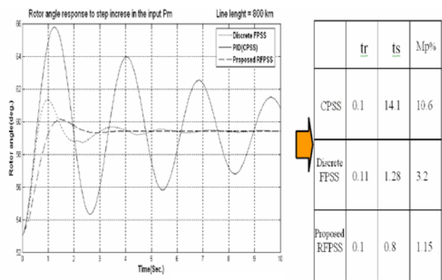
Fig. 8-b L=800 km
