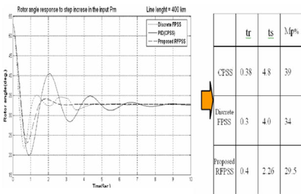
Fig. 8-a L=400 km
