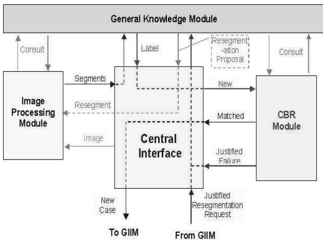
Fig. 2 The IISM Module
