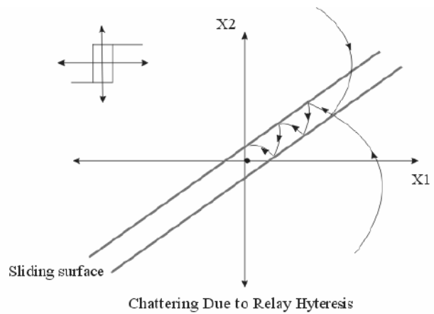
Fig. 6 Chattering phenomenon.
