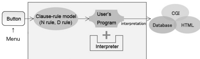
Fig. 10. Interpreter
