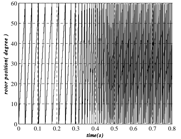
Fig. 3 Actual and desired rotor position for 30-150 rad/s
